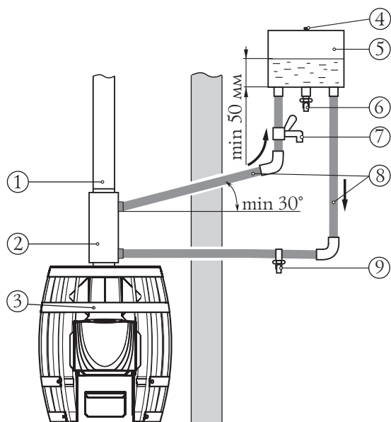
Paveikslėlis 8. Vandens kaitinimo sistemos montavimo schema su «virdulio» tipo šilumokaičiu «Kostakan»
