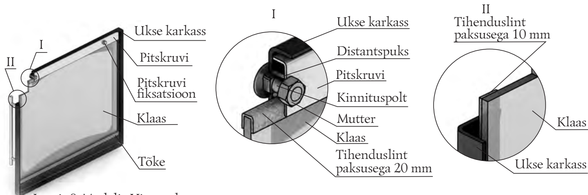
Joonis 9. Mudeli «Vitra» ukse valgusläbilaskva ekraani kinnitus
